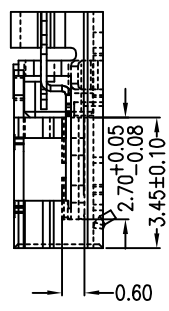
SEC A-A
